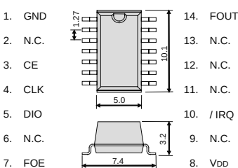
SOP - 14 pin
