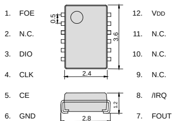
VSOJ - 12pin
